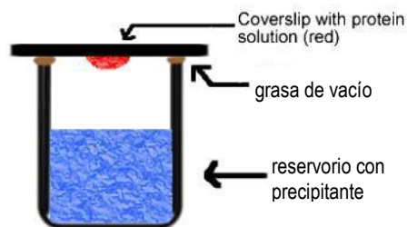
Figura 7. Método de difusión de vapor de la gota colgante para cristalización de proteínas. (Rhodes, Gale. Crystallography Made Crystal Clear . San Diego: Academic Press, 1993)
